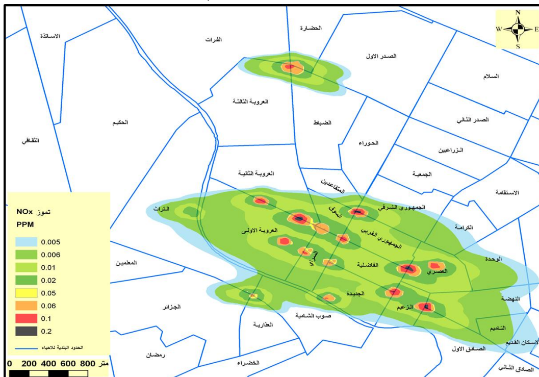
خريطة رقم(7) تراكيز اكاسيد النتروجين NOx في انبعاثات التقاطعات للذروة الصباحية خلال شهر تموز لسنة 2017(EARMOD view 8.9.0) (ARC GIS 10.4
