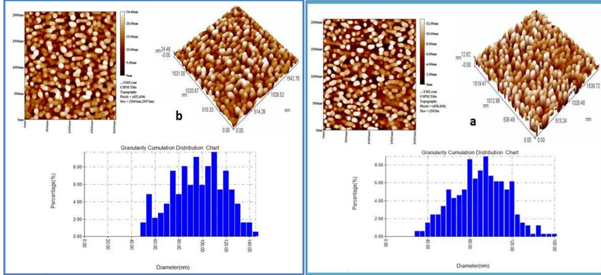
شكل (3): صور AFM ببعدين (2D) و ثلاثة ابعاد (3D) ومخطط التوزيع الاحصائي لمعدلات الحجوم الحبيبية
