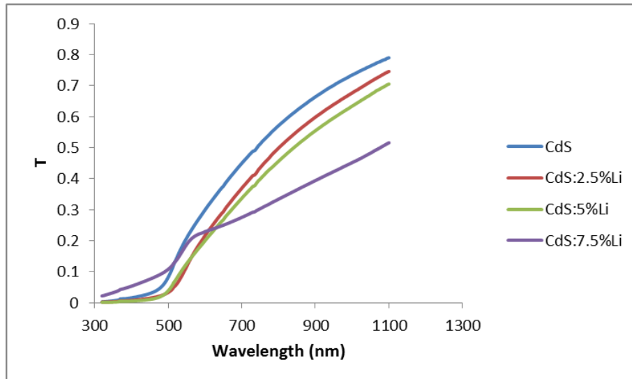
شكل (4): النفاذية لأغشية CdS النقية والمشبوبة ب Li
