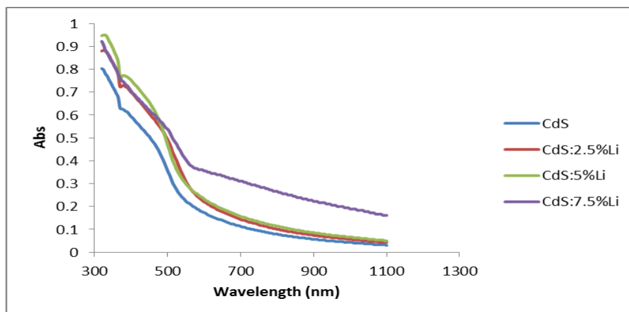
شكل (5): الامتصاصية لأغشية CdS النقية والمشوبة بالليثيوم (Li)
