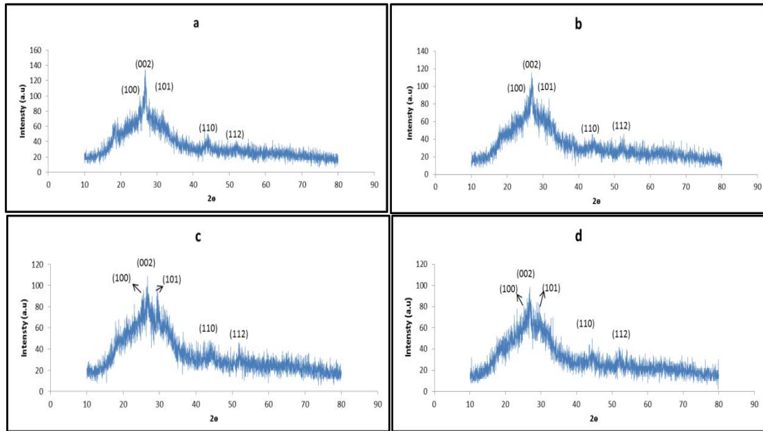
شكل (1): حيود الاشعة السينية CdS:a CdS:2.5%Li:b CdS:5%Li:c CdS:7.5%Li:d
