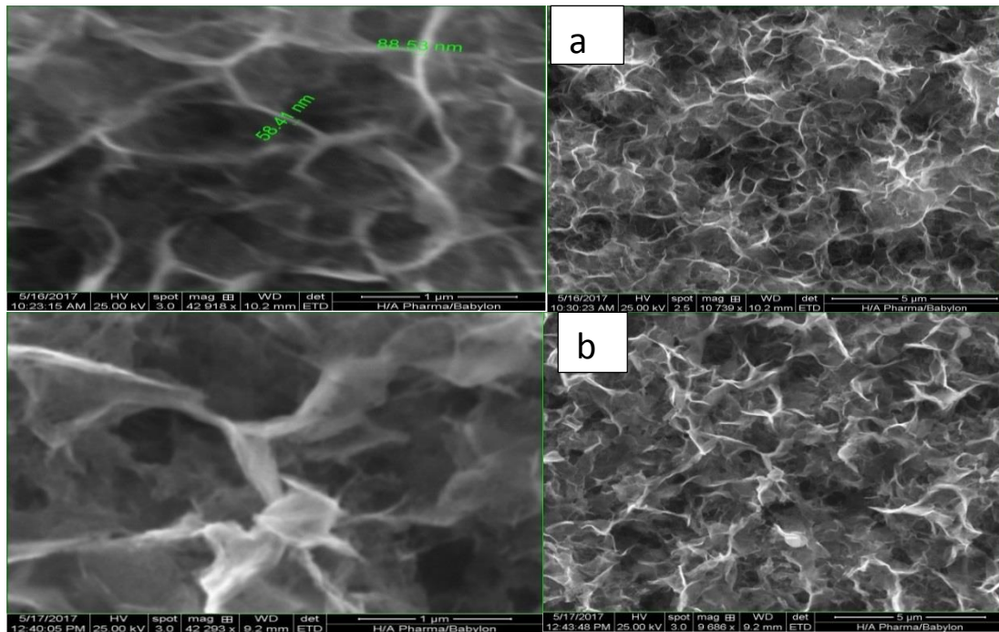
شكل (2) : صور المجهر الالكتروني الماسح (SEM) CdS :a CdS:7.5%Li :b
