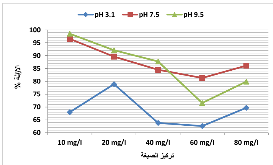
شكل ( ٢ ) تأثير تركيز الصبغة على نسبة إزالة الصبغة عند زمن الاتزان وقيم مختلفة من pH و ١ غم من CKD .
